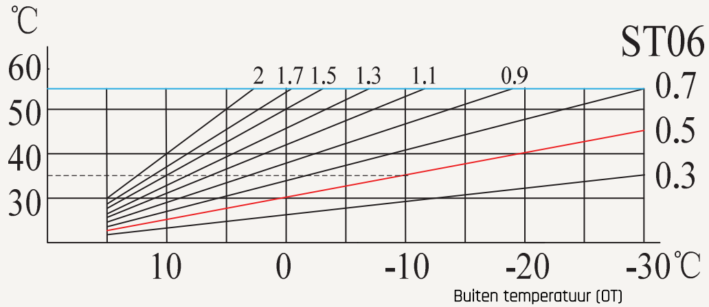
Figuur 8.5 – Stooklijn ( ST02 = 20^{\circ}C ): regelt temperatuur T (verwarmen) t.o.v. buitentemperatuur ( OT ) voor verschillende ST06 -waarden.
