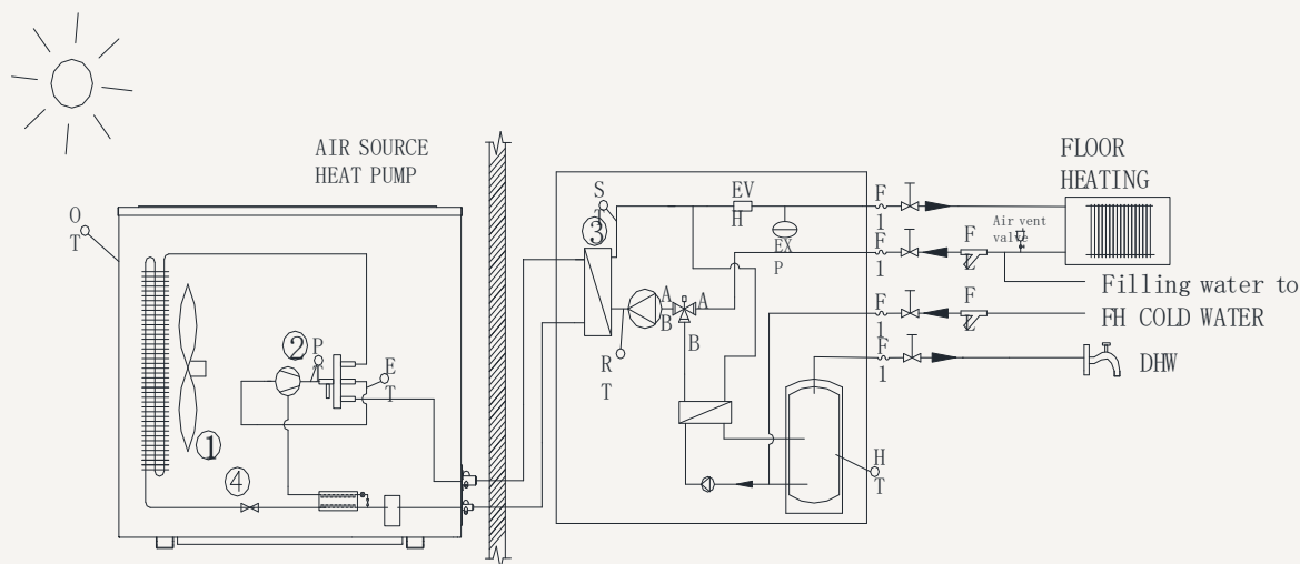
Figuur 1.1 – Koudemiddelcircuit en werkingsprincipe. ① luchtwarmtewisselaar (verdamer) · ② compressor · ③ platenwisselaar (condensor) · ④ expansieventiel. Labels in de tekening: FLOOR HEATING = vloerverwarming, COLD WATER = koud water, DHW = warm tapwater, Filling water to FH = vulwater verwarmingscircuit.
