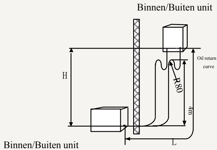
Figuur 6.2 – Oliebocht bij hoogteverschil (oil return curve) – H = hoogteverschil, L = leidinglengte.
