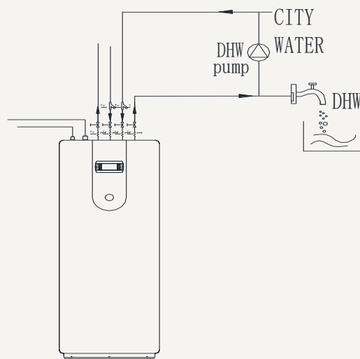
Figuur 6.7 – Aansluiting tapwatercirculatiepomp. CITY WATER = leidingwater · DHW pump = tapwaterpomp.
